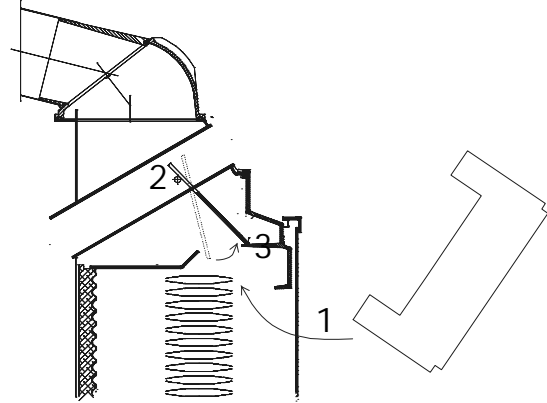
Fig. 7: Einlegen der oberen Zugumlenkplatte
