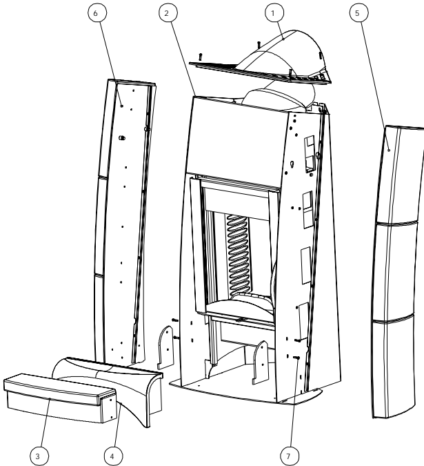
Fig. 6: Verkleidungsteile
