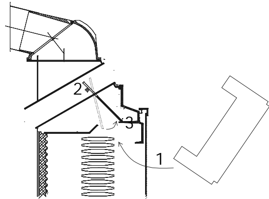
Fig. 7: Insertion de la plaque supérieure de déviation de tirage
