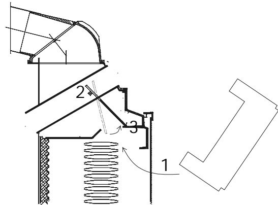
Fig. 7: Inserimento del deflettore superiore
