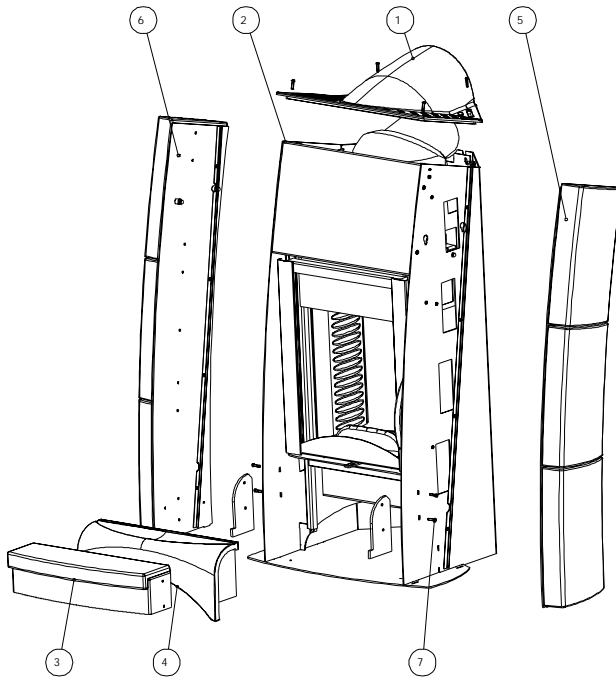
Fig. 6: Parties d'habillage
